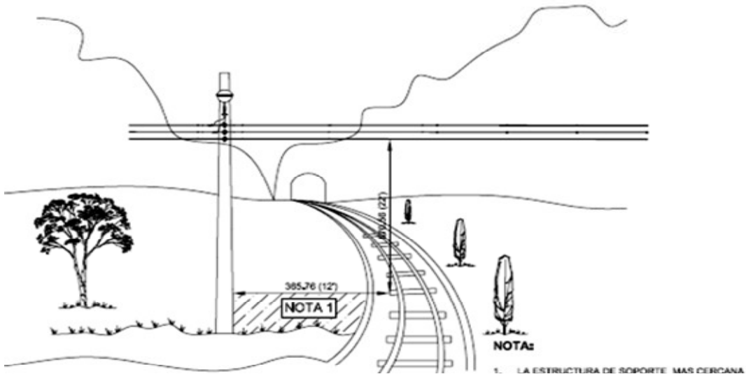
Figura #2. Debe existir una distancia mínima horizontal de 3.85 m (12') de cualquier parte de la estructura de soporte más cercana a la vía férrea, cuando los conductores cruzan o están paralelos a las vías férreas, a una altura no menor de 6.70 m (22').
