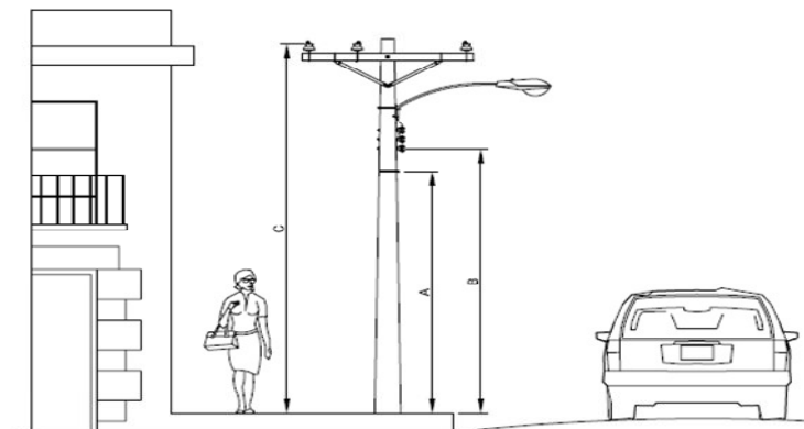
Figura #3. Distancia mínima vertical donde los alambres, cables y conductores pasan a lo largo y dentro de los límites de carreteras u otros derechos de paso, pero no sobresalen del camino.
