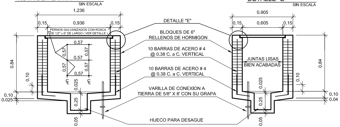
SECCION "A"
