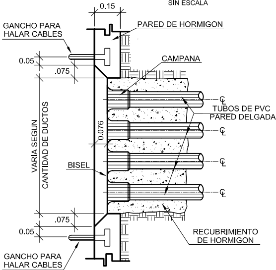
DETALLE DE VENTANA PARA DUCTOS
