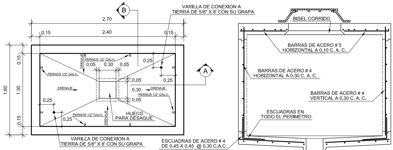
LOSA INFERIOR (PLANTA) SIN ESCALA
