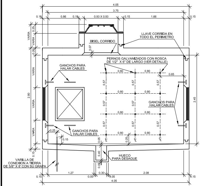
SECCION "B" SIN ESCALA
