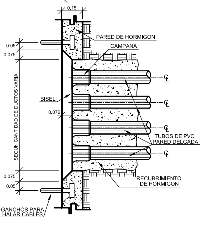
DETALLE DE VENTANA PARA DUCTOS SIN ESCALA
