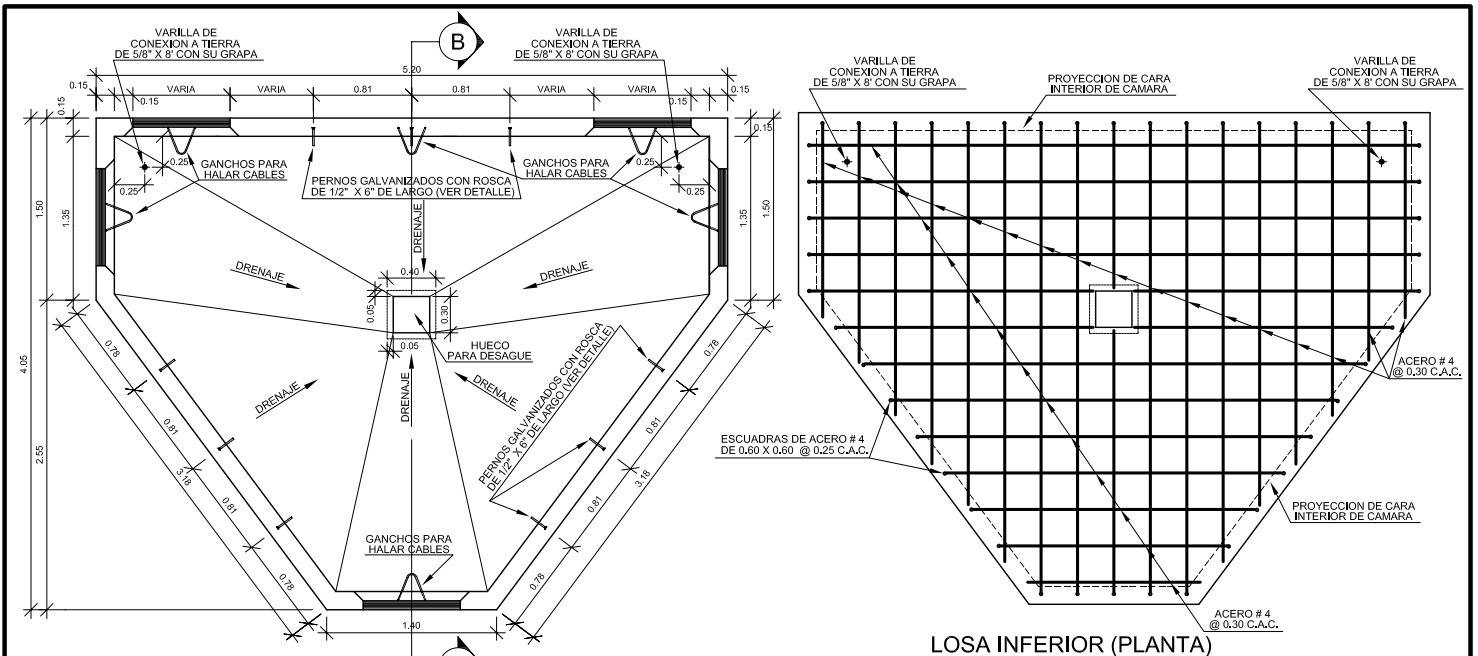
VISTA DE PLANTA SIN ESCALA
