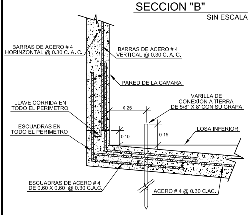
DETALLE "N" SIN ESCALA
