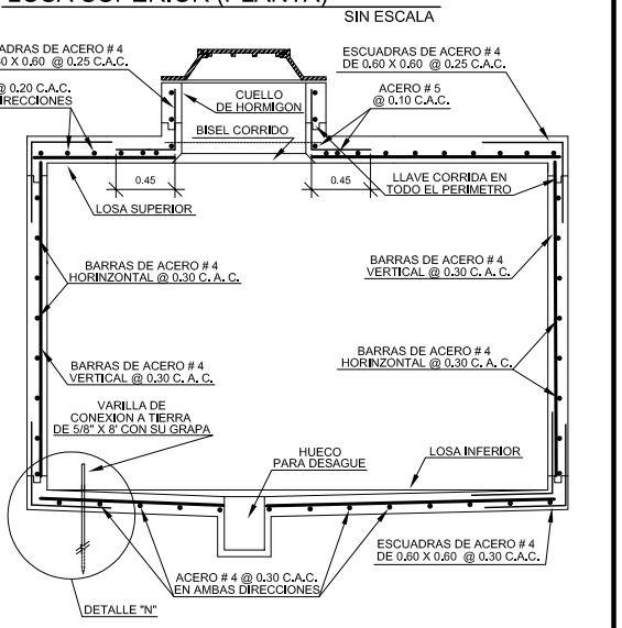
SECCION "A" (ESTRUCTURAL) SIN ESCALA
