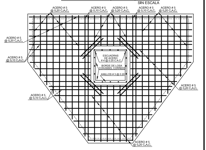
LOSA SUPERIOR (PLANTA)
