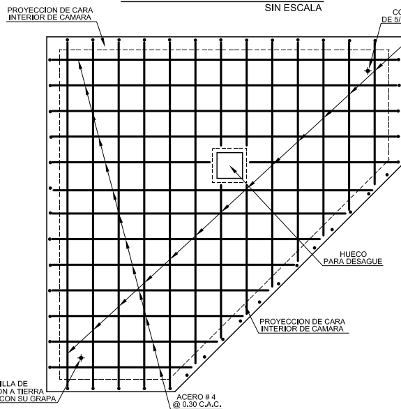
LOSA INFERIOR (PLANTA) SIN ESCALA
