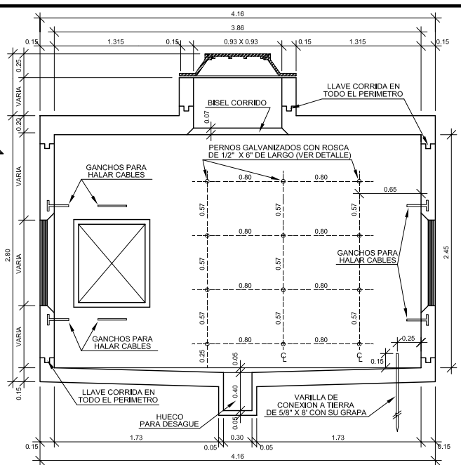
SECCION "B"
