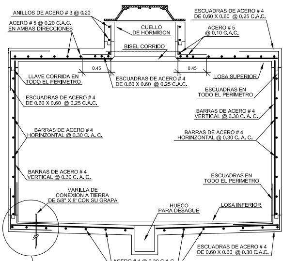
SECCION "A" (ESTRUCTURAL) SIN ESCALA
