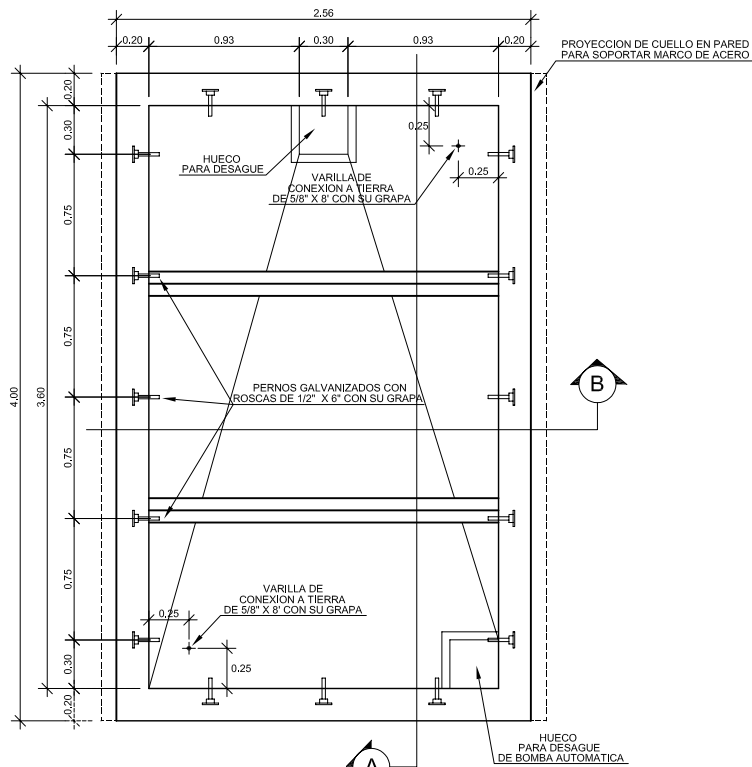
LOSA INFERIOR (PLANTA) SIN ESCALA
