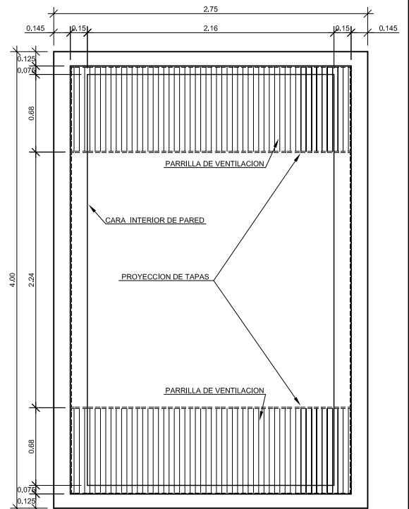
LOSA SUPERIOR (DISTRIBUCION DE TAPAS) SIN ESCALA
