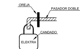
DETALLE "N" SIN ESCALA
