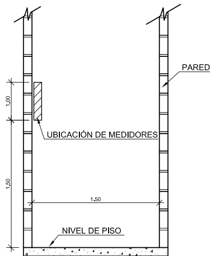
SECCION "A" SIN ESCALA
