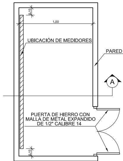
VISTA DE PLANTA SIN ESCALA
