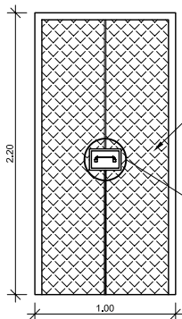
PUERTA DE HIERRO SIN ESCALA
