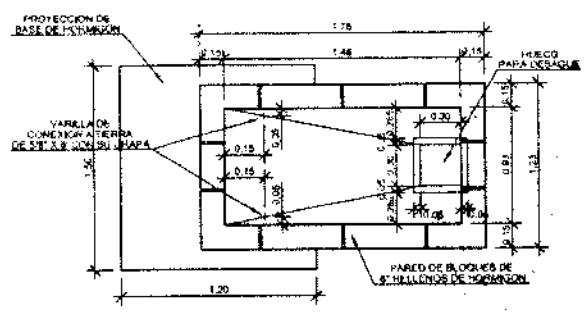
LOSA INFERIOR (PLANTA) SIN ESCALA
