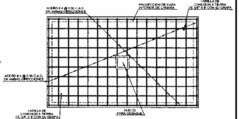
LOSA INFERIOR (PLANTA) SIN ESCALA
