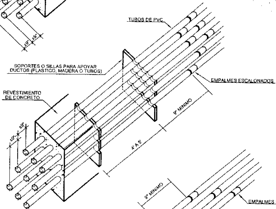
FIGURA 2 ESCALONAMIENTO VERTICAL DE LAS HILERAS
