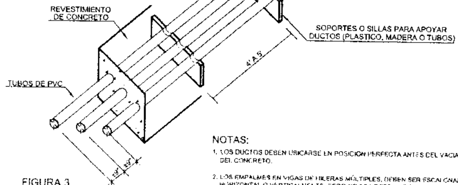
FIGURA 3 VIGADUCTO DE UNA HILERA
