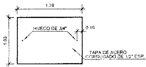
DETALLE DE TAPA DE ACERO SIN ESCALA
