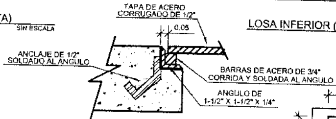
DETALLE S-1 SIN ESCALA
