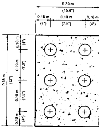
SECCION "D"
