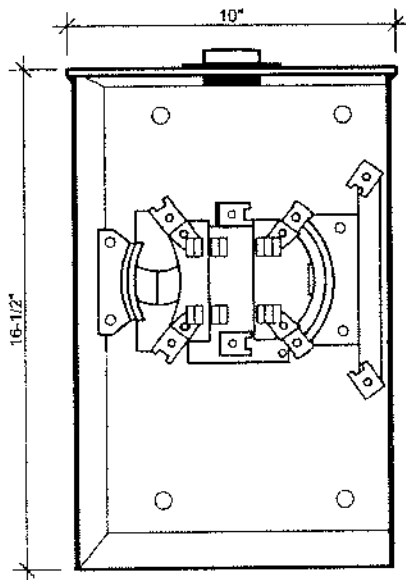
200 AMPERE - 7 TERMINALES
