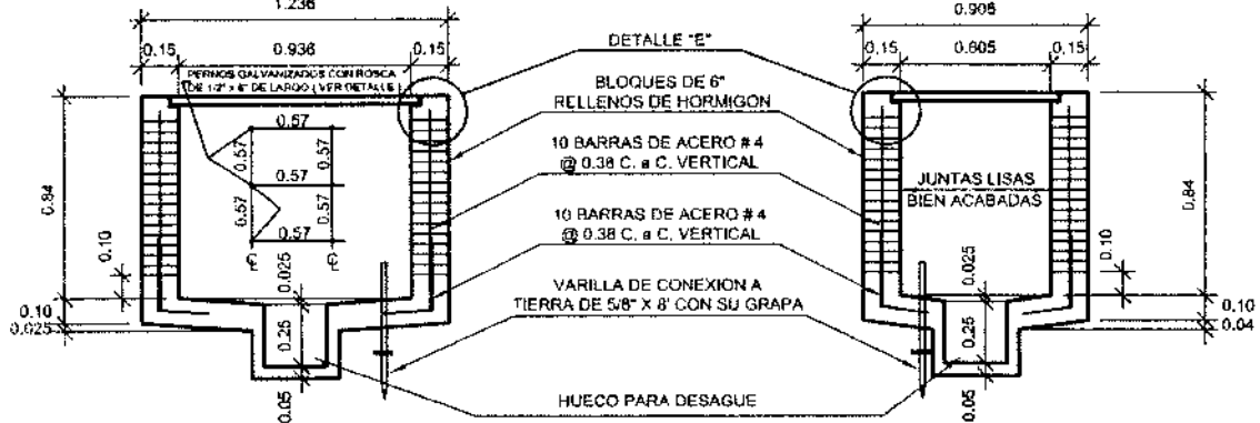
SECCION "A" SIN ESCALA
