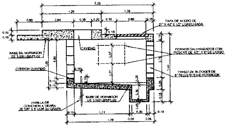
SECCION "A" SIN ESCALA
