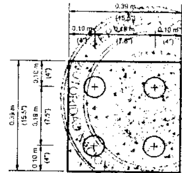
SECCION "C"
