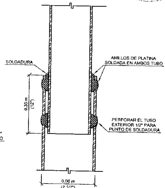
DETALLE "B" SIN ESCALA
