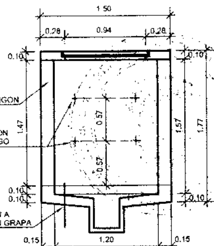
SECCION "B" SIN ESCALA
