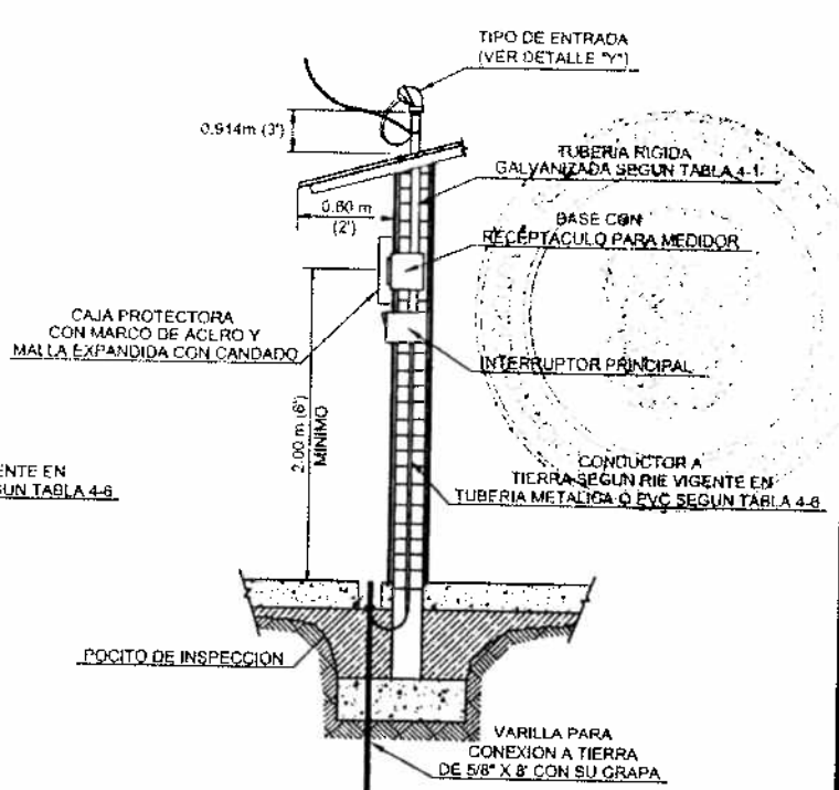
ALTERNATIVA "B" SIN ESCALA
