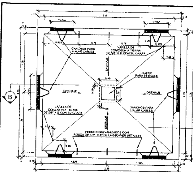
VISTA DE PLANTA SIN ESCALA
