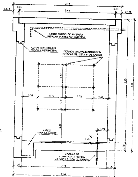
SECCION B-B SIN ESCALA
