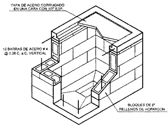
ISOMETRICO SIN ESCALA
