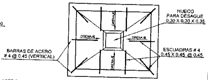
LOSA INFERIOR (PLANTA) SIN ESCALA
