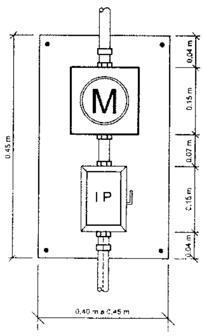
DETALLE "A" SIN ESCALA
