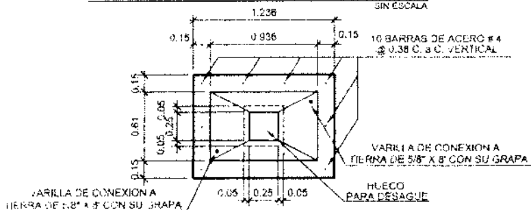
LOSA INFERIOR (PLANTA) SIN ESCALA
