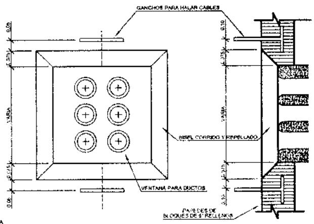
DETALLE TÍPICO PARA VENTANAS DE DUCTOS SIN ESCALA
