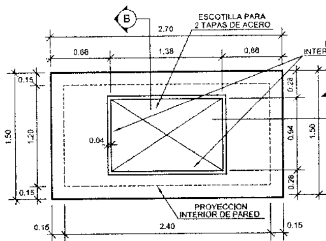
LOSA SUPERIOR (PLANTA) SIN ESCALA
