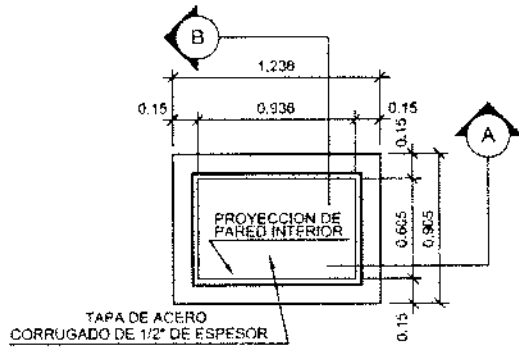
VISTA DE PLANTA SIN ESCALA
