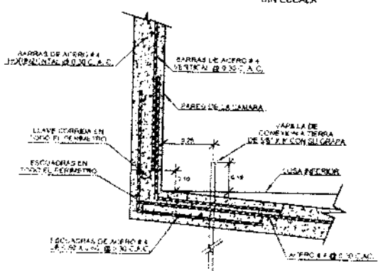
DETALLE "N" SIN ESCALA
