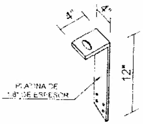
DETALLE "X" EN PARED
