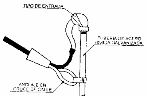
DETALLE "Y" EN PARED
