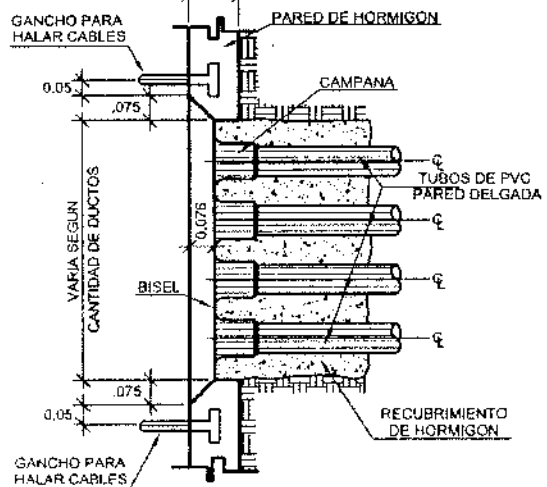
DETALLE DE VENTANA PARA DUCTOS SIN ESCALA
