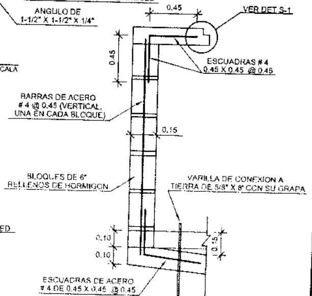
SECCION ESTRUCTURAL SIN ESCALA
