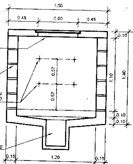
SECCION "X" SIN ESCALA
