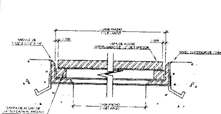
SECCION "A" SIN ESCALA
