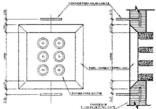
DETALLE TIPOICO PARA VENTANAS DE DUCTOS SIN ESCALA
