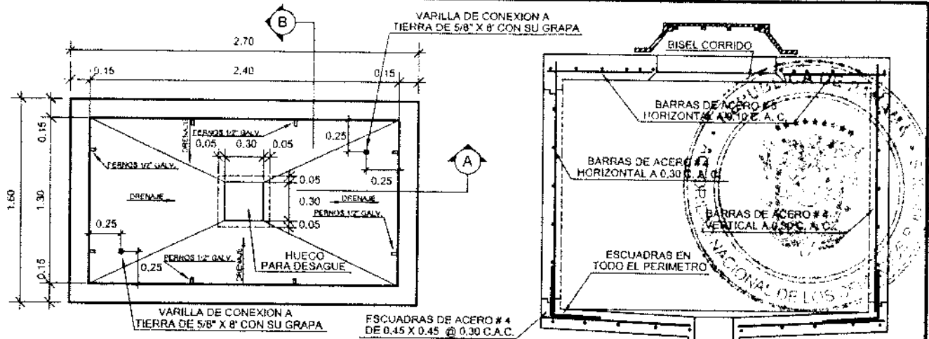
LOSA INFERIOR (PLANTA)
