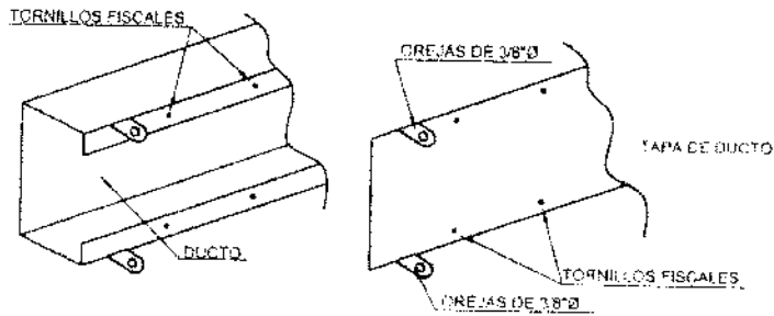
DETALLE "A" LINEA A-A
