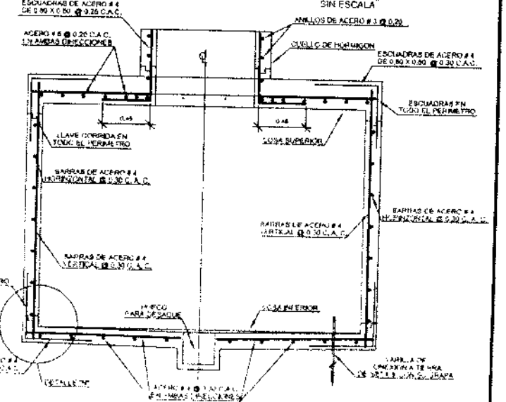
SECCION "A" (ESTRUCTURAL) SIN ESCALA
