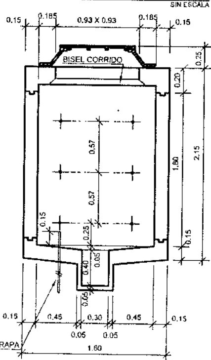
SECCION "B"
