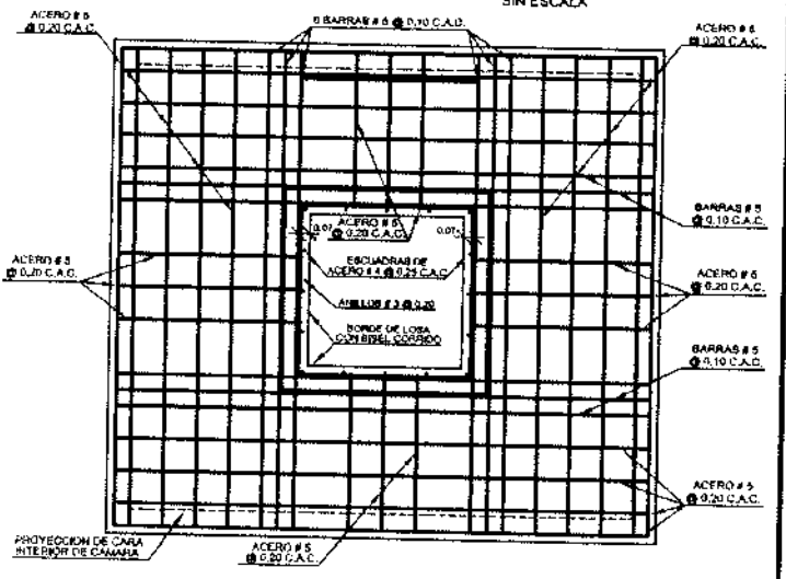
LOSA SUPERIOR (PLANTA) SIN ESCALA
