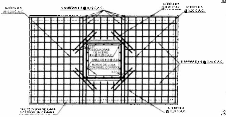
LOSA SUPERIOR (PLANTA) SIN ESCALA
