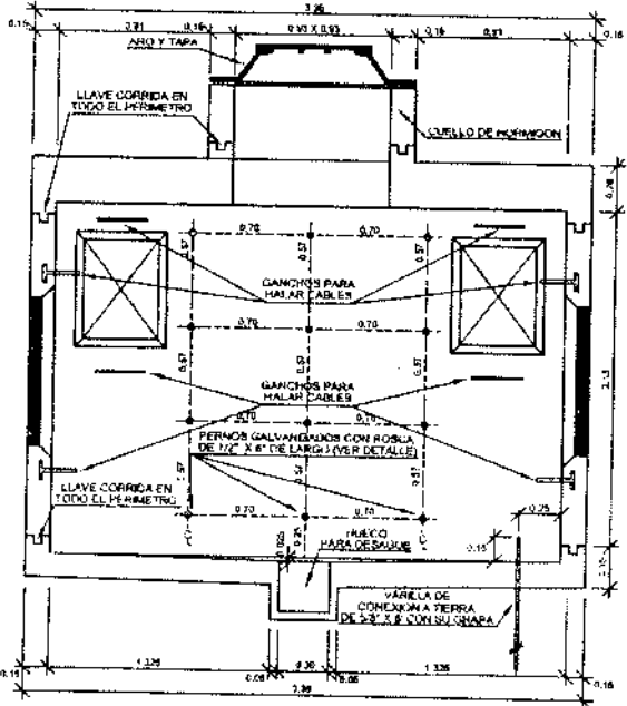
SECCION "B" SIN ESCALA
