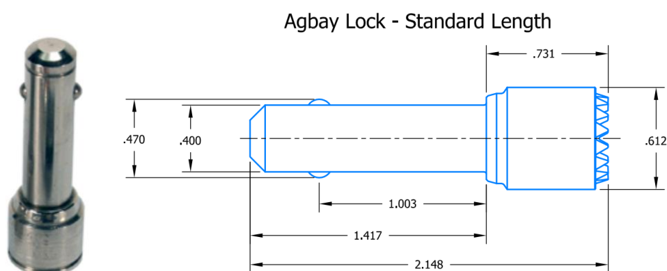
Figura.1 Dimensiones del Tornillo de cierre tipo barril.
