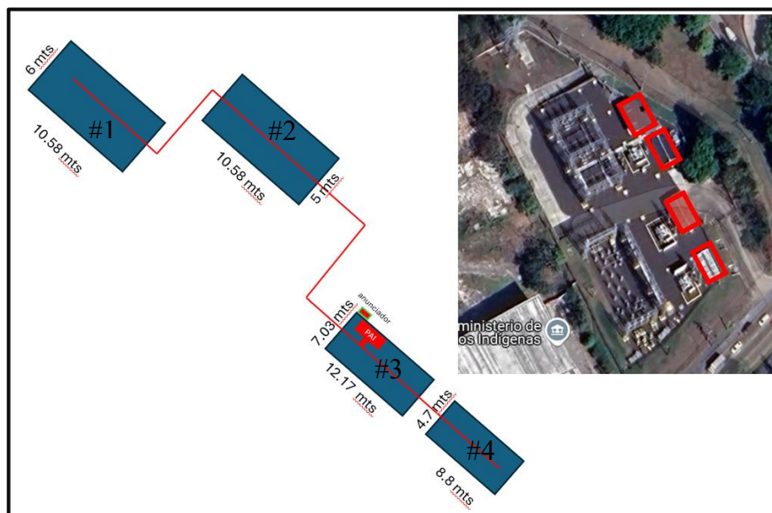
Imagen 1. subestación Sta. Maria, en el lado derecho. Esquema ilustrativo de donde debe quedar el nuevo panel de alarma de incendio y en cual caseta, en el lado izquierdo. Adicional, longitudes aproximadas de las casetas de la subestación.
