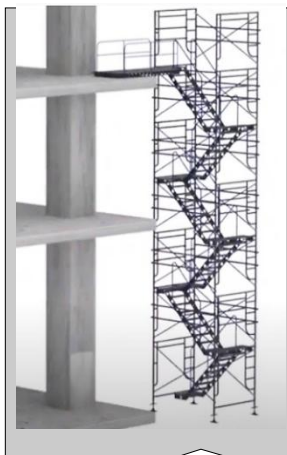
Torre de escalera de andamios
